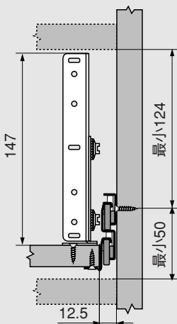
キャビネット最小寸法
