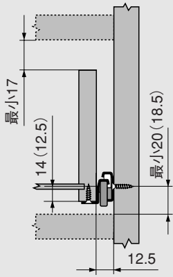
キャビネット最小寸法 230M (230E)
