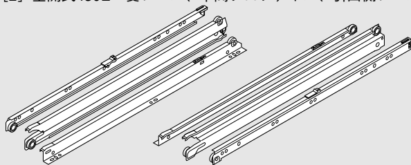
[2] 全開式430E 受レール、中間プロファイル、引出側レールのセット
