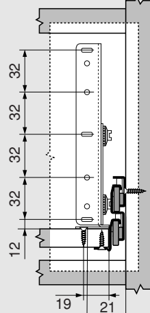
引出前板取付寸法
