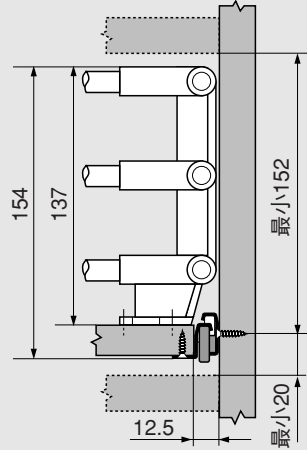
キャビネット最小寸法 3段ギャラリ付
